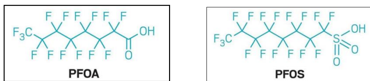
Fig. 1 : Formules structurales des PFOA & PFOS
